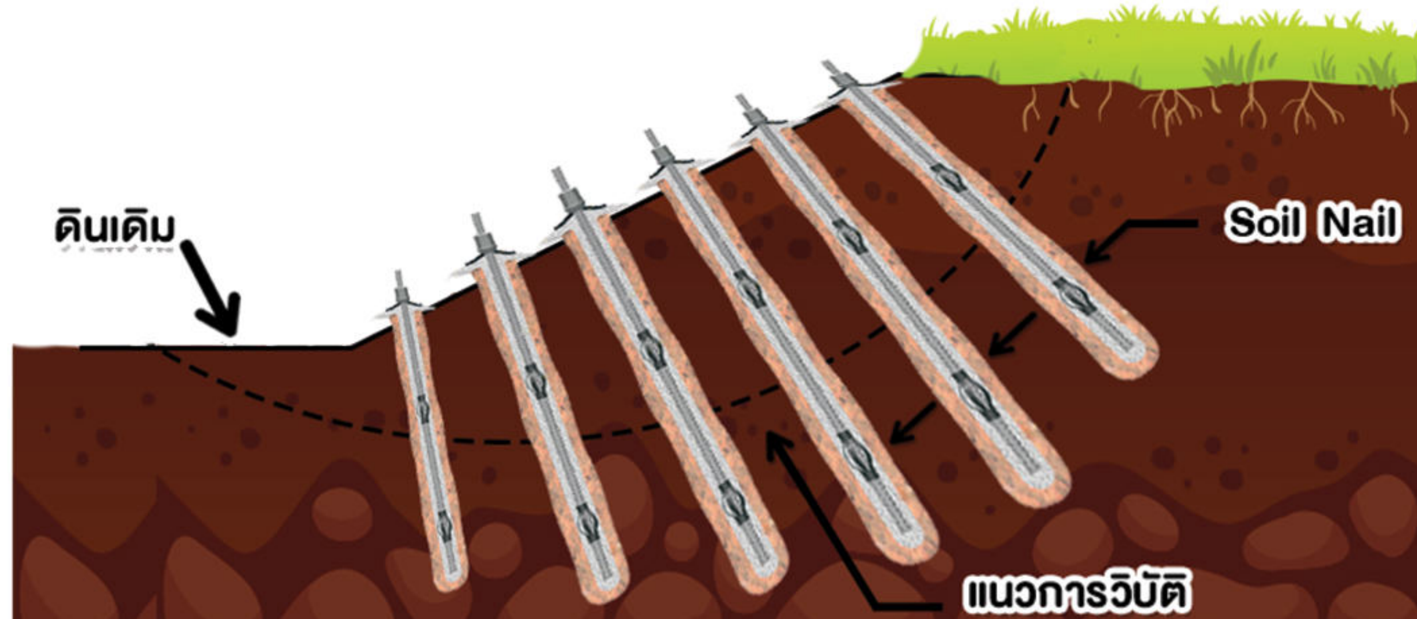
ตัวอย่างการเสริมความแข็งแรงให้ดินโดยใช้ Soil Nail
